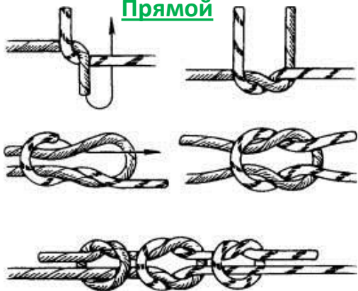
Прямой
